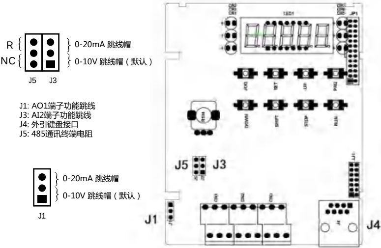
图 3-6 跳线及辅助端子位置示意图
