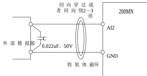
图 3-8 模拟量输入端子处理接线图
