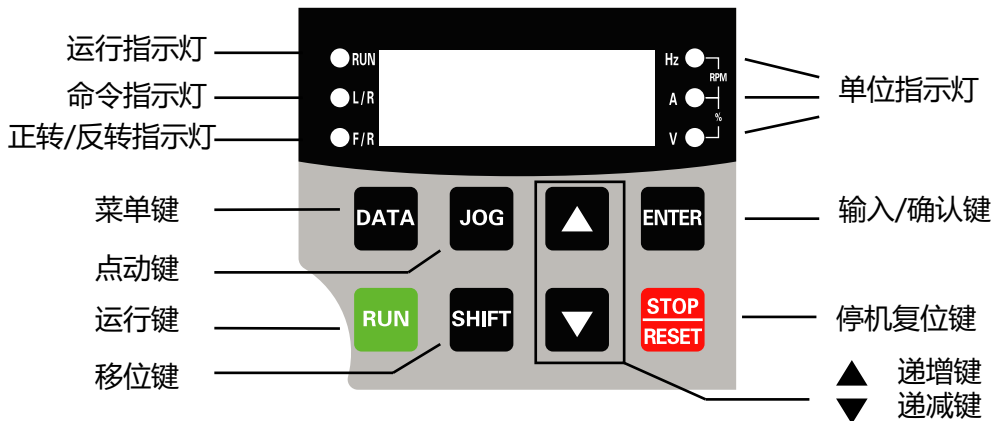
图 4-1 操作面板示意图
