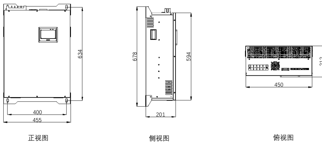
图 5 100A、75A 壁挂模块尺寸
