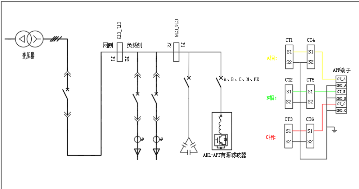
图 14 电流互感器安装位置及 SN-APF 电流互感器做“减法”接线示意图
