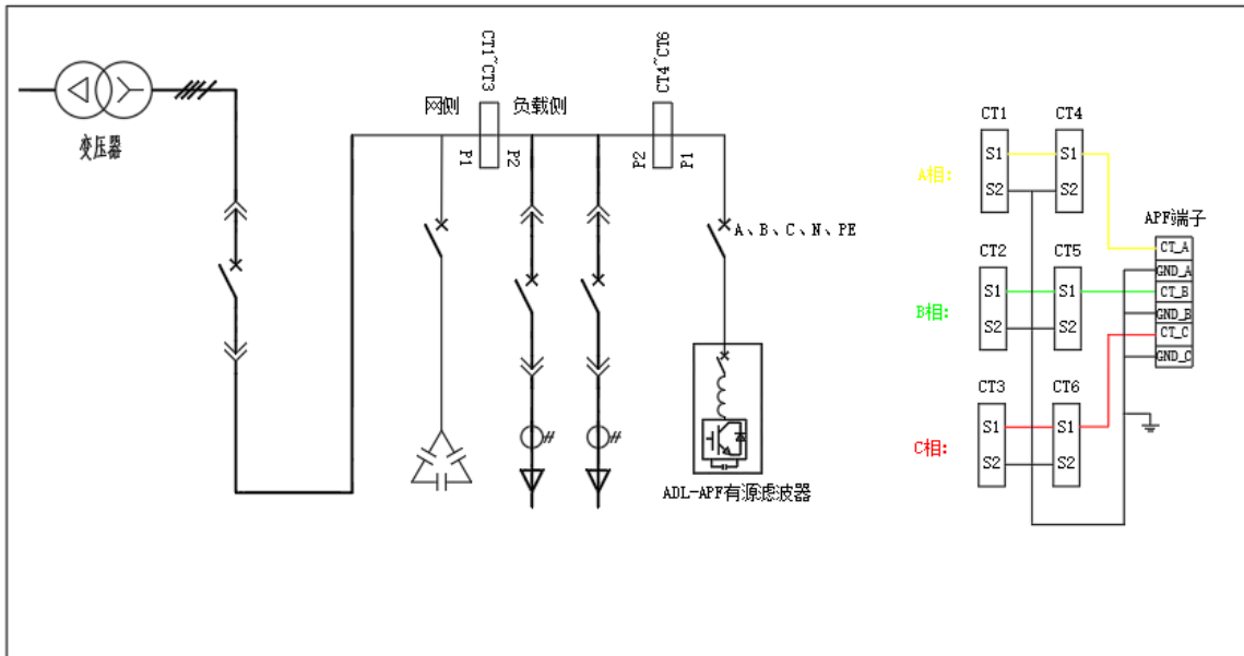
图 13 电流互感器安装位置及 SN-APF 电流互感器做“减法”接线示意图
