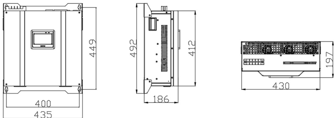
图 7 50A、30A 壁挂模块尺寸
