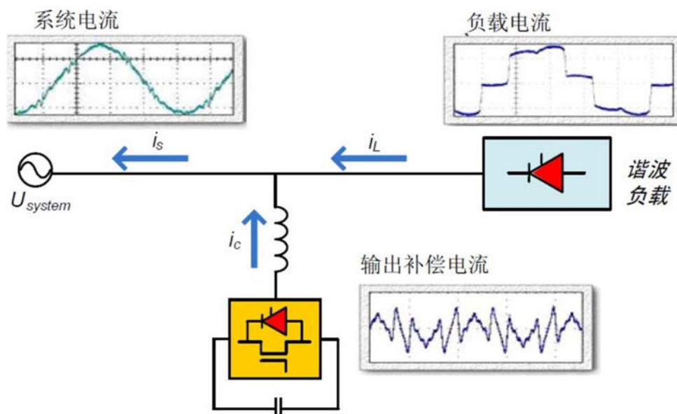
图 1 SN-APF 基本原理
