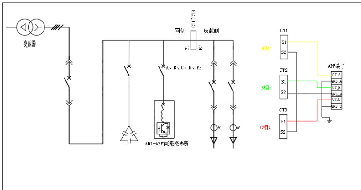
图 11 电流互感器安装位置及单台 SN-APF 电流互感器接线示意图
