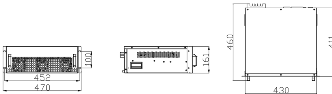
图 6 50A、30A 抽屉模块尺寸
