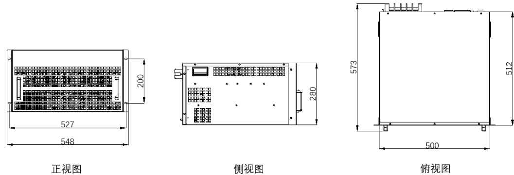
图 2 150A 抽屉模块尺寸
