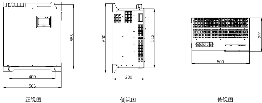
图 3 150A 壁挂模块尺寸
