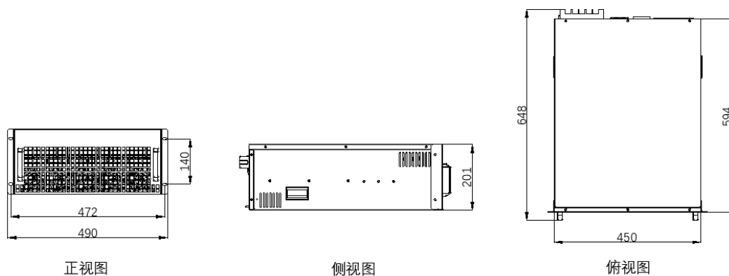
图 4 100A、75A 抽屉模块尺寸
