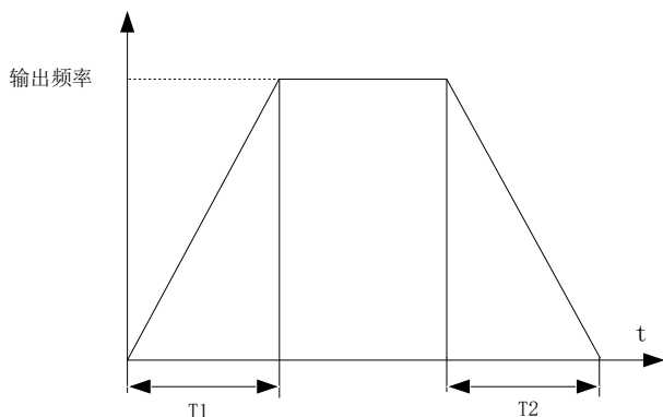
图 7-18 直线加减速示意图
