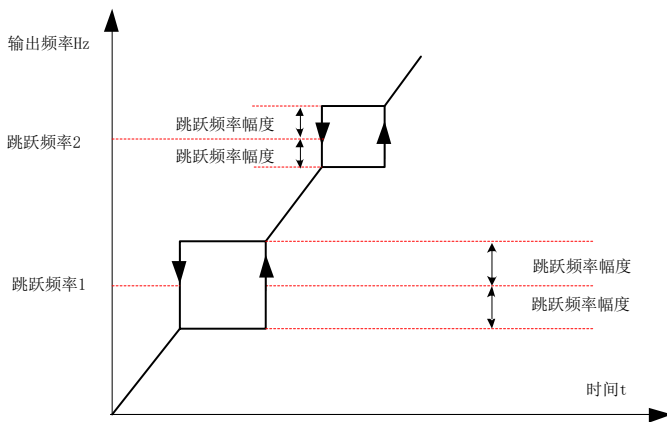
图 7-20 跳跃频率及范围示意图
