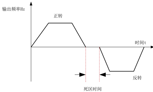
图 7-21 正反转死区时间示意图
